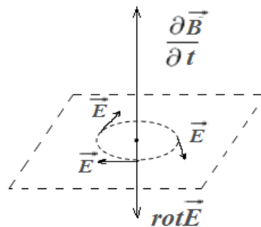
Рис 9. Связь \frac{\partial \vec{B}}{\partial t} и \text{rot } \vec{E}
