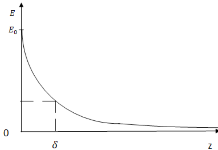
Рис. 43. График убывания поля
