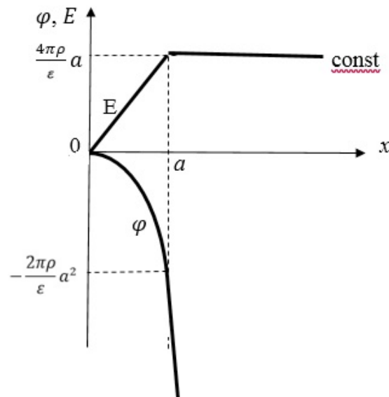
Рис. 59. Потенциал и напряженность электрического поля «Великой китайской стены»
