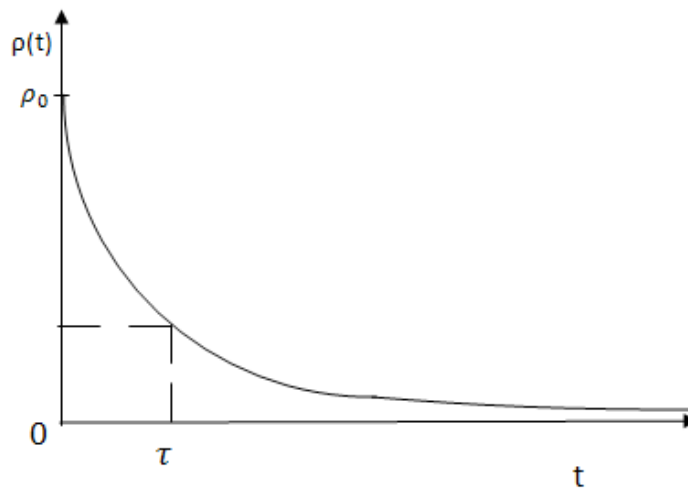
Рис. 41. График убывания плотности заряда в проводнике
