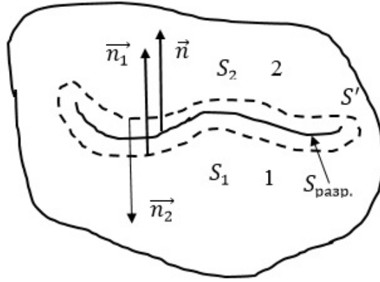
Рис. 38. Поверхности в окрестности \vec{n}
