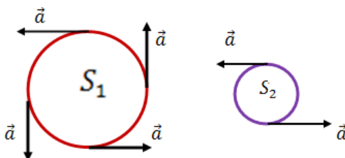
Рис. 51. К понятию поверхностной циркуляции
