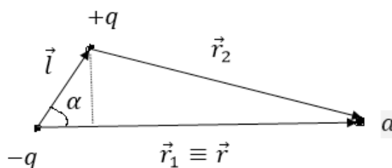
Рис. 21. Диполь. К расчету потенциала \varphi
