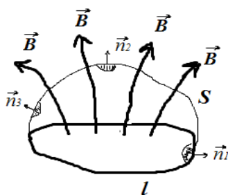
Рис. 8. Поток вектора \vec{B} через поверхность S
