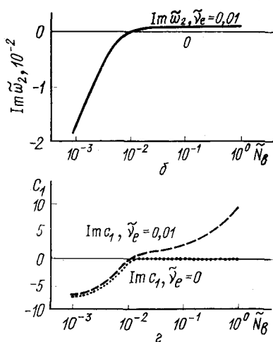
Рис. 16.4. Зависимости величины, характеризующей линейное затухание (а, б), коэффициентов связи плазменных (в, г) и пучковых (д) волн от плотности пучка (сплошные кривые на рис. 16.4, г, д отвечают гидродинамическому приближению; гидродинамические и кинетические значения на рис. 16.4, в совпадают); \bar{k}_0 = -0,93 \cdot 10^{-3} ; \bar{u}_b = 15 ; \bar{V}_{0b} = 7,7 \cdot 10^2
