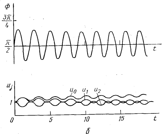
рис. 10.1, б. Если же какие-либо два из углов \theta_{ij} отличаются в точности на \pi (рис. 10.2, а), то получается предельно устойчивое решение, пример которого показан на рис. 10.2, б. Наконец, при
