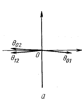
Рис. 10.2. Конфигурация векторов \exp(i\theta_{ij}) в случае, когда два угла \theta_{ij} отличаются в точности на \pi (а), и вид решения при фазовых углах, изображенных на рис. 10.2, а для v_j=0,01 (б)
