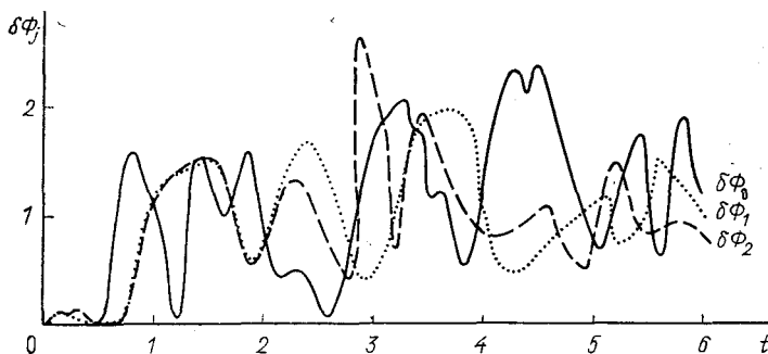
Рис. 18.7. Временная эволюция первоначально малого разброса фаз волн из пакета 0 при условии, что начальный разброс фаз волн из пакетов 1 и 2 равен нулю
