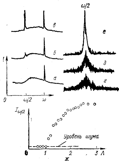
Рис. 23.1. Нелинейный распадный спектр:
