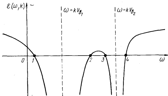
Рис. 10.4. Общий вид диэлектрической проницаемости \varepsilon(\omega, k) при фиксированном k в случае холодной двухпотоковой системы со скоростями V_{b1} и V_{b2} .
