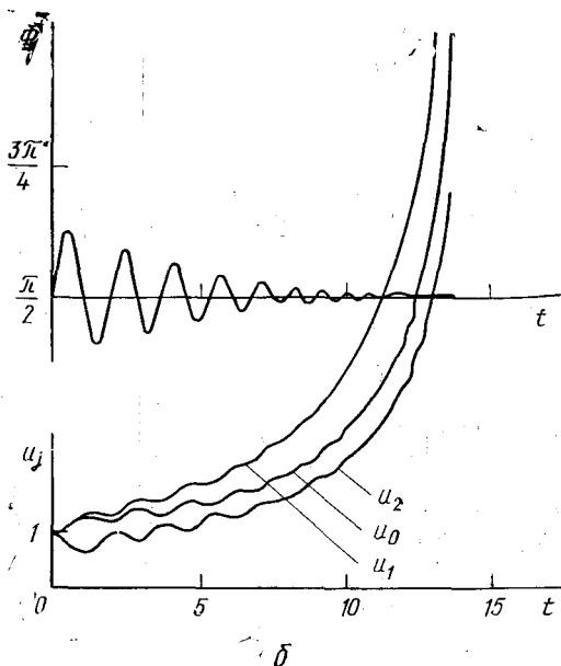
рис. 10.1, б. Если же какие-либо два из углов \theta_{ij} отличаются в точности на \pi (рис. 10.2, а), то получается предельно устойчивое решение, пример которого показан на рис. 10.2, б. Наконец, при
