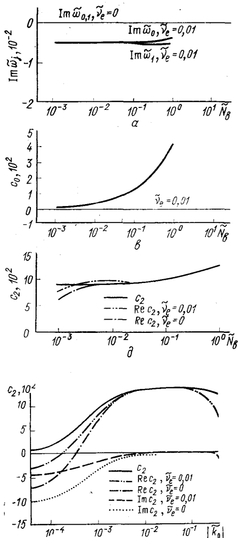
Рис. 16.5. Зависимость коэффициента связи пучковой волны от волнового числа плазменной волны |\bar{k}_0| (сплошная кривая рассчитана в гидродинамическом приближении); N_b = 10^{-3} , \bar{u}_b = 15 , \bar{V}_{0b} = 7,7 \cdot 10^2
