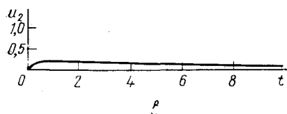
Рис. 12.3. Временная зависимость величины u_2 = -(1/2) dy/dt , где y — решение уравнения (12.24) при \rho=1 (а), \rho=2 (б) и \rho=5 (в)
