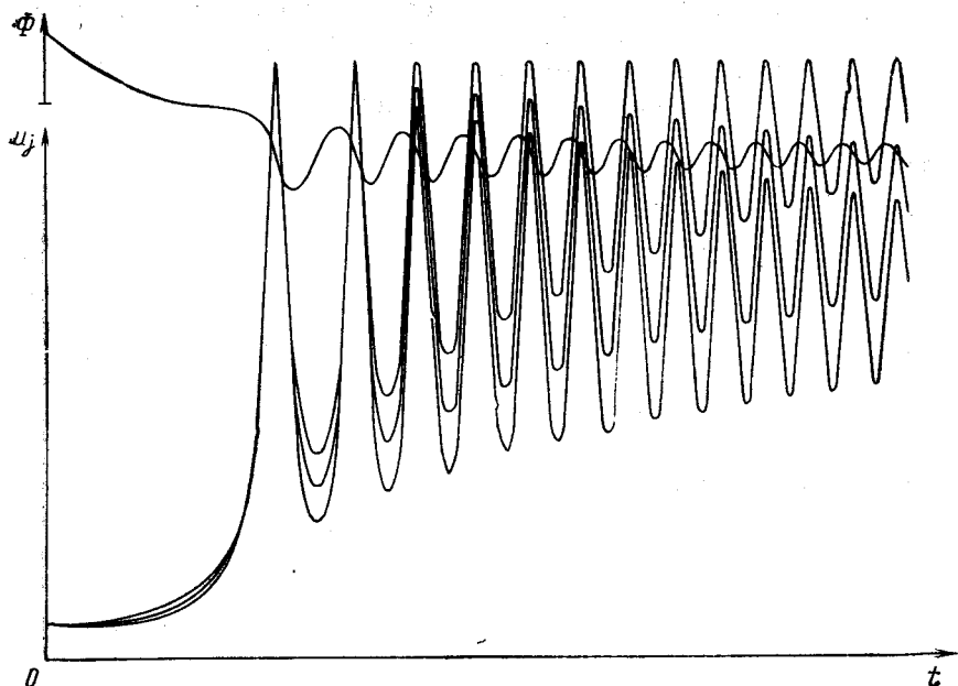
Рис. 15.3. Временная зависимость амплитуд u_j и фазы \Phi при v_0=0,1 , v_1=0,2 и v_2=0,3 (начальные значения всех амплитуд равны)
