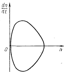
Рис. 9.5. Взаимодействие трех волн с энергией одного знака на фазовой плоскости ( s=-1 , n=u_j^2 )
