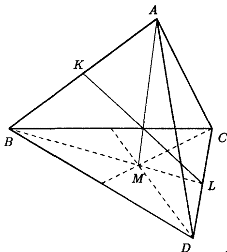
рис.3. Тетраэдр
