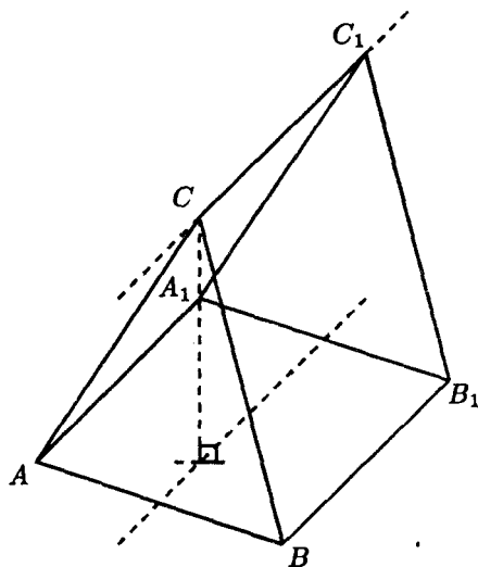
рис.14. Треугольная призма.
