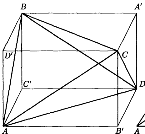
рис.9. Прямоугольный параллелепипед описан около равногранного тетраэдра.
