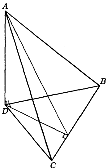
рис.7. Прямоугольный тетраэдр.
