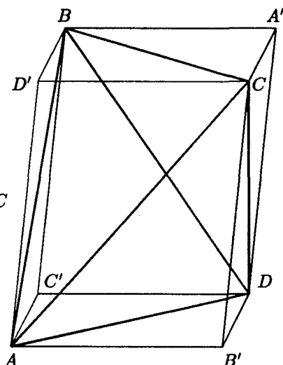
рис.4. Описанный параллелепипед.
