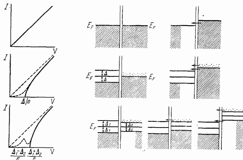
Рис. 99. Туннельный эффект через оксидную пленку между двумя нормально или сверхпроводящими твердыми телами. Верхний ряд. Если оба тела — нормальные проводники, то в равновесии зона проводимости заполнена до энергии E_F . При приложении к ним напряжения происходит сдвиг химического потенциала (энергии Ферми) одного проводника по отношению к другому. В результате пойдет ток, вольтамперная характеристика которого имеет вид прямой линии. Средний ряд. Если одно из тел — сверхпроводник, то при T = 0 ток возникает только тогда, когда химический потенциал нормального проводника увеличится на величину \Delta . При T \neq 0 , из-за теплового возбуждения электронов слабый ток возникает при напряжении, меньшем \Delta . Нижний ряд. Если граничат два сверхпроводника, то при T = 0 ток возникает только при напряжении, равном \Delta_1 + \Delta_2 . При T \neq 0 возникает дополнительный ток, который при \Delta_1 - \Delta_2 имеет максимум.
