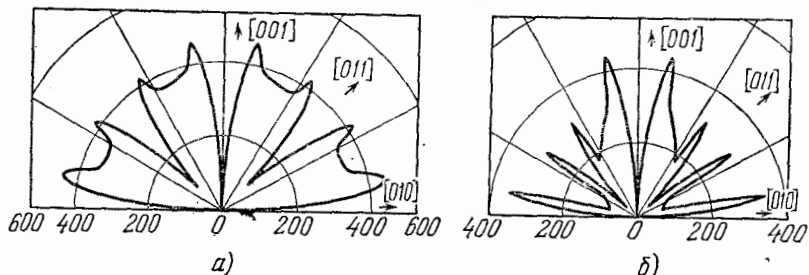
Рис. 64. Изменение поперечного сопротивления в магнитном поле \Delta R/R_0 у меди при 18 000 Гс и 4,2 К как функция ориентации направления тока по отношению к кристаллическим осям: а) магнитное поле направлено по [100], б) магнитное поле отклонено от направления [100] менее чем на 3^\circ . (По И. Р. Клаудеру и И. Е. Кунцлеру [46].)
