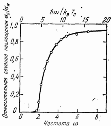
Рис. 97. Край поглощения сверхпроводника (индий). Фотоны поглощаются только тогда, когда они обладают энергией 2\Delta , достаточной для разрушения куперовской пары. (По Блэкмору [4].)
