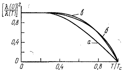
Рис. 101. Глубина проникновения магнитного поля по теории БКШ ( a —локальное приближение, б —нелокальное приближение) и ( в ) по эмпирическому закону \lambda^{-2} \sim 1 - (T/T_c)^4 . (По Феттеру и Валечка [79].)
