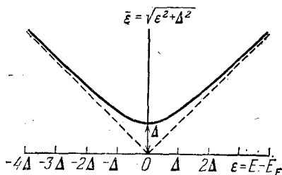
Рис. 95. Энергия \bar{\varepsilon} квазичастиц, которые описывают возбужденное состояние сверхпроводящего электронного газа.
