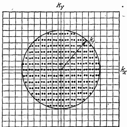
Рис. 1. Сфера Ферми радиуса k_F в \mathbf{k} -пространстве. Каждый элемент объема размером (2\pi)^3/V_g содержит два состояния. При T=0 эти состояния внутри сферы Ферми заняты электронами с противоположно направленными спинами.
