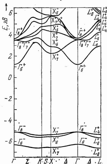
Рис. 79. Зонная структура йодистого калия. (По Оверхофу (Phys. Stat. Sol. (b) 43, 575, 1971).)
