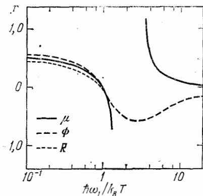
Рис. 66. Показатель степени r в степенном законе \tau \sim E^r времени релаксации для электрон-ЛО-фононного взаимодействия. Эффективные времена релаксации для подвижности \mu , термо-Э.Д.С. \Phi и постоянной Холла R , полученные вариационным методом, приблизительно совпадают при высоких и низких температурах. В этом случае предположение о существовании единого времени релаксации представляется обоснованным. (По Эренрайху (J. Appl. Phys. 32, 2155, 1961).)
