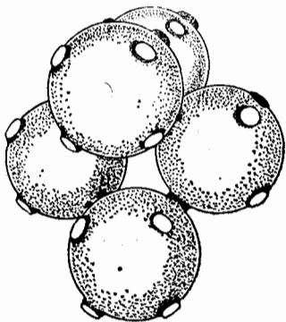
Рис. 33. Поверхности Ферми у меди в повторяющейся зонной схеме. (По Макинтошу [56].)
