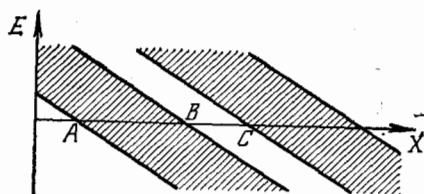
Рис. 26. Если к энергии зонной модели прибавить электростатическую энергию постоянного электрического поля, то зоны на диаграмме зависимости E от x оказываются наклонными. Электрон, перемещающийся из A в B , будет либо отражен обратно в зону, либо в результате туннельного эффекта переброшен в следующую, более высокую зону.
