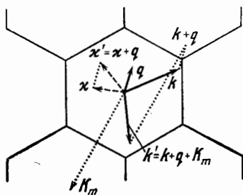
Рис. 58. Нормальные процессы ( k' = k + q ) и процессы переброса ( k' = k + q + K_m ) в Brillouin-зоне плоской гексагональной решетки.
