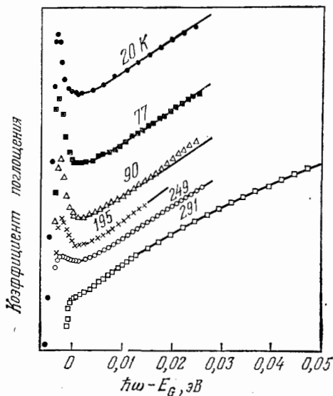
Рис. 75. Экситонные линии перед краем прямого поглощения в германии. Линии, как это особенно ясно видно при низких температурах, переходят в континуум. При высоких температурах экситонные добавки исчезают. (По Мак-лину [39].)
