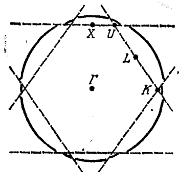
Рис. 31. Сфера Ферми у алюминия проходит через вторую, третью и четвертую зоны Бриллюэна. Ее форма слегка искажена по сравнению со случаем свободных электронов только вблизи брэгговского отражения. (По Харрисону [10].)
