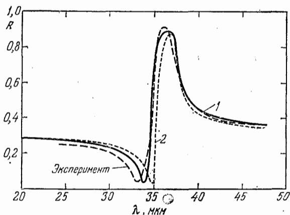
Рис. 90. Коэффициент отражения для GaAs и две теоретические кривые отражения 1 и 2, полученные подгонкой параметров \epsilon_0 , \epsilon_\infty , \omega_t и \gamma . (По Эренрайху (Phys. Rev. 120, 1951, 1960).)
