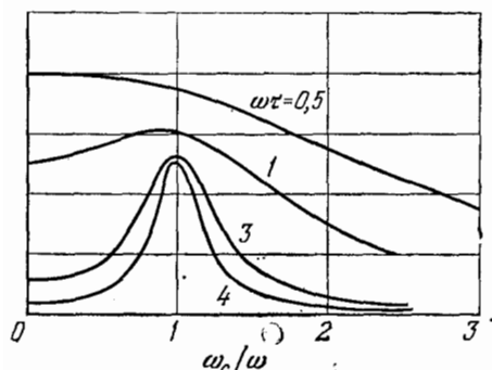
Рис. 85. Поглощение в окрестности циклотронно-резонансной частоты \omega_c . При отсутствии электрон-фононного взаимодействия ( \omega_0 = 1/\tau = \infty ) кривая поглощения есть \delta -функция от \omega = \omega_c . С увеличением электрон-фононного взаимодействия вершина кривой поглощения, по уравнению (75.18), уплощается.
