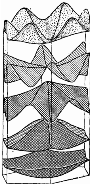
Рис. 23. Зоны рис. 21, б «сглаженные» влиянием слабого потенциала решетки.
