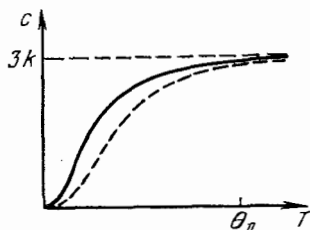
Рис. 45. Теплоемкость в приближении Дебая (сплошная кривая) и в приближении Эйнштейна (пунктирная кривая).
