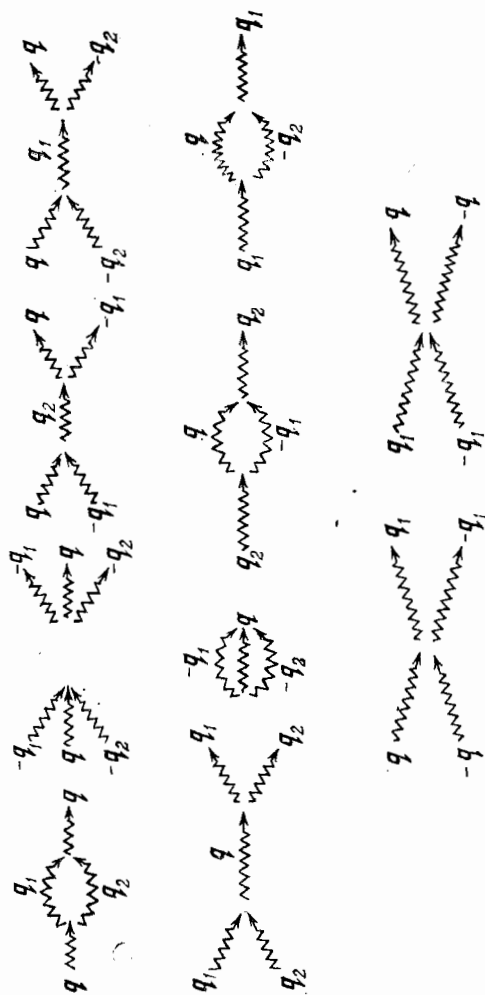
Рис. 103. Фонон-фононные процессы, которые ведут к перенормировке фононной энергии
