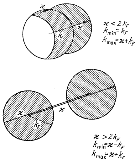
Рис. 2. Переходы электронов из сферы Ферми при заданном добавочном импульсе k . Области внутри сферы Ферми, из которых могут осуществляться переходы, и области вне сферы Ферми, в которые электроны могут переходить, заштрихованы.
