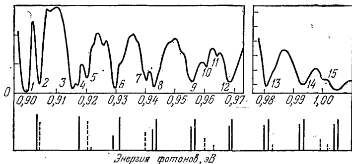
Рис. 84. Сравнение спектра поглощения на рис. 83 с теорией для E \parallel V . Наверху — экспериментальный спектр, внизу — вычисленные энергии перехода. Сплошные линии — переходы из зоны тяжелых дырок (верхняя валентная зона), пунктирные линии — переходы из зоны легких дырок (нижняя валентная зона). Высота линий соответствует теоретической интенсивности. (По Рот, Лэксу и Цвердлингу (Phys. Rev. 114, 90, 1959).)
