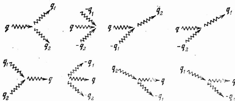
Рис. 102. Диаграммы трехфоновых процессов взаимодействия. В процессах первого ряда один фонon q исчезает; в процессах второго ряда один фонon q возникает.
