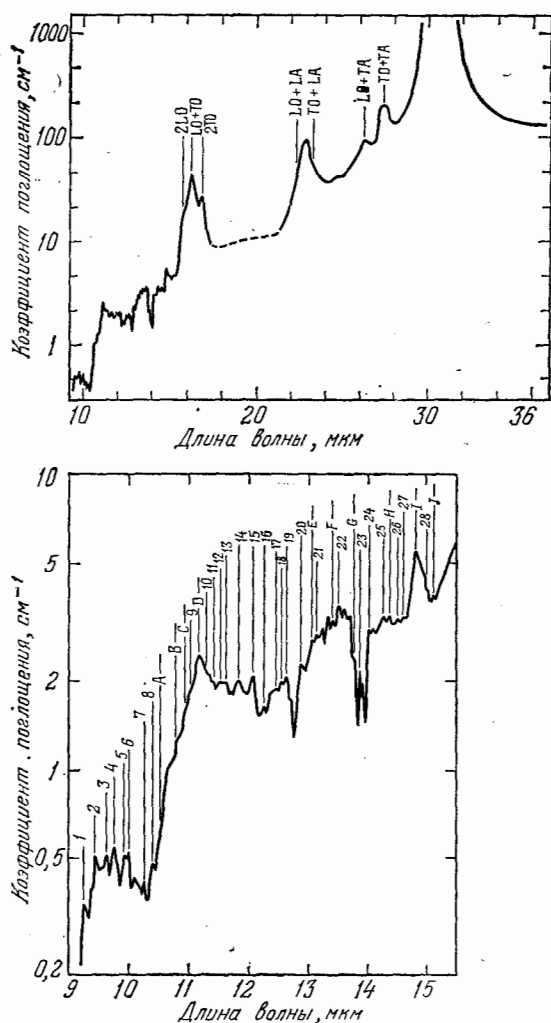
Рис. 91. Многофононные спектры для AlSb и сопоставление структур для двухфононных процессов (верхний рисунок) и трех- и четырехфононных процессов (нижний рисунок). (По Джонсону [111,9].)
