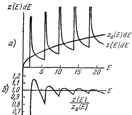
Рис. 8. а) Зависимость плотности состояний от энергии для B=0 и B \neq 0 . б) Отношение числа состояний ниже некоторой заданной энергии в магнитном поле к числу состояний без магнитного поля.
