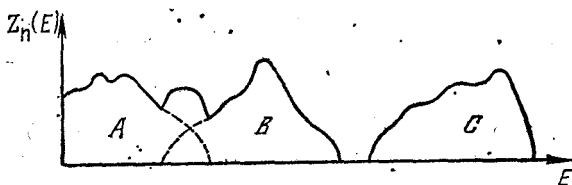
Рис. 27. Плотность состояний (схематически) для перекрывающихся зон и для зон, разделенных запрещенной зоной.
