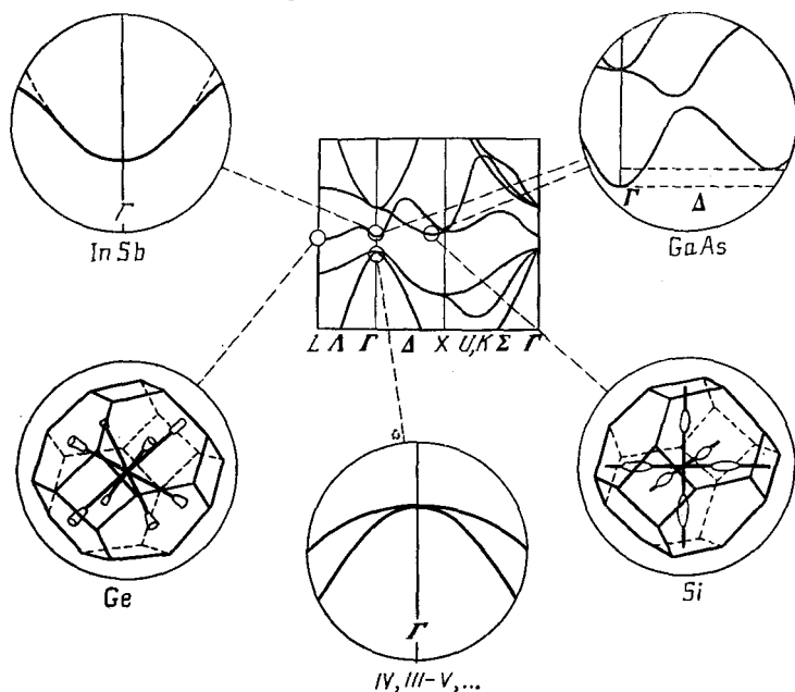
Рис. 39. Важнейшие детали зонной структуры полупроводника.
