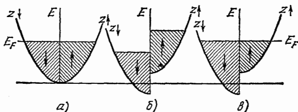
Рис. 10. Спиновый парамагнетизм Паули. В магнитном поле к кинетической энергии электрона, в зависимости от направления спина, добавляется энергия \pm \mu_B B . Тогда ниже энергии Ферми E_F лежит большее число состояний с одним направлением спина, чем с обратным. На рисунке приведены плотности состояний, в зависимости от энергии, раздельно для обоих направлений спина; занятые состояния заштрихованы: а) без магнитного поля, б) смещение состояний в магнитном поле, в) занятые состояния в магнитном поле после установления равновесия.
