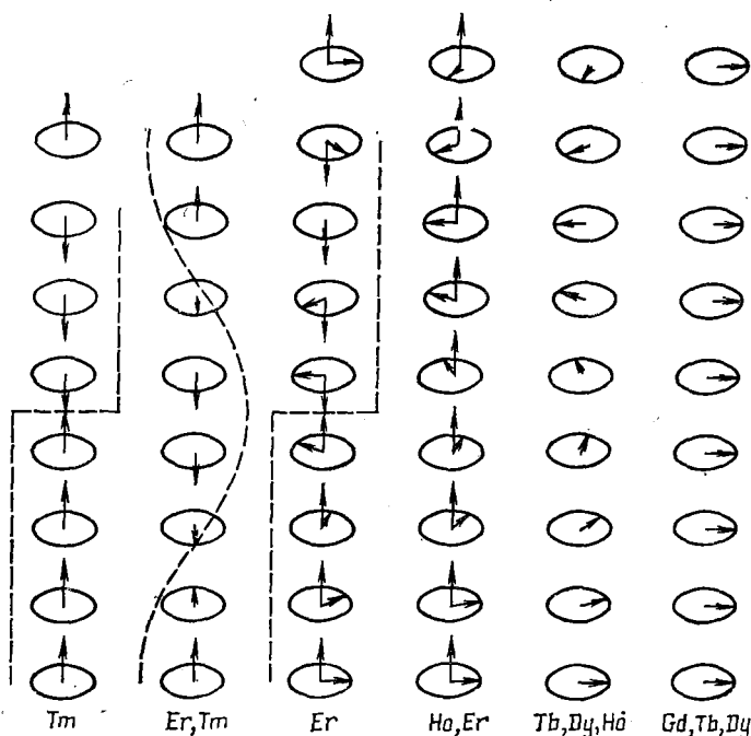
Рис. 53. Расположение спинов вдоль оси z в слоистых решетках редких земель. (По Куперу [57.21].)
