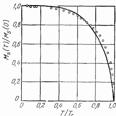
Рис. 52. Намагничивание насыщения по уравнению (40.8) и сравнение с экспериментальными данными у никеля. (По Киттелю [12].)
