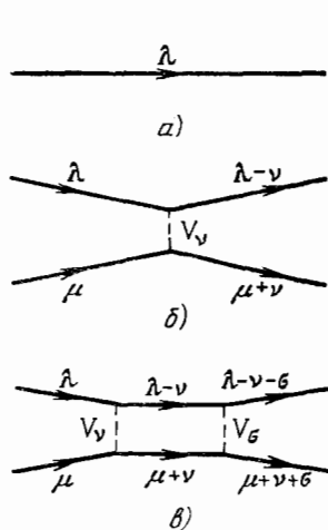
Рис. 12. Диаграммы электрон-электронного взаимодействия: а) невзаимодействующего электрона с импульсом k_\lambda , б) взаимодействие между двумя электронами, при котором происходит обмен импульсом k_\nu , в) два следующие друг за другом взаимодействия б).
