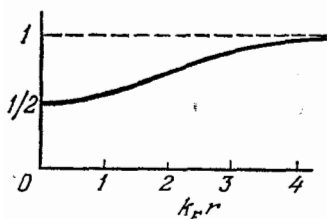
Рис. 11. Обменная дырка электрона в приближении Хартри—Фока (см. (11.8)).
