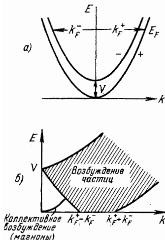
Рис. 56. а) Смещение состояний свободных электронов с одним направлением спинов на величину обменной энергии V относительно состояний с другим направлением спинов. б) Наряду с возбуждением одного электрона из сферы Ферми с сохранением спина при переходе, спин может перевернуться. Это возможно, только если между энергией и импульсом при возбуждении существует соотношение, которое попадает в область, заштрихованную на рисунке. Спиновые волны могут распасться на эти элементарные возбуждения, если их энергия лежит выше граничной энергии, необходимой для возбуждения. Для аналогичного случая ср. с рис. 15. (По Эллиотту [39]).
