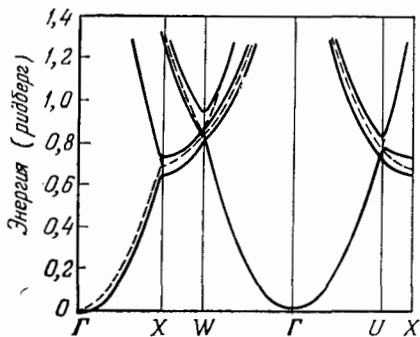
Рис. 30. Валентные зоны алюминия. (По Харрисону [10].)
