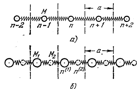
Рис. 43. Линейная цепочка: а) с одним атомом и б) с двумя атомами в ячейке.
