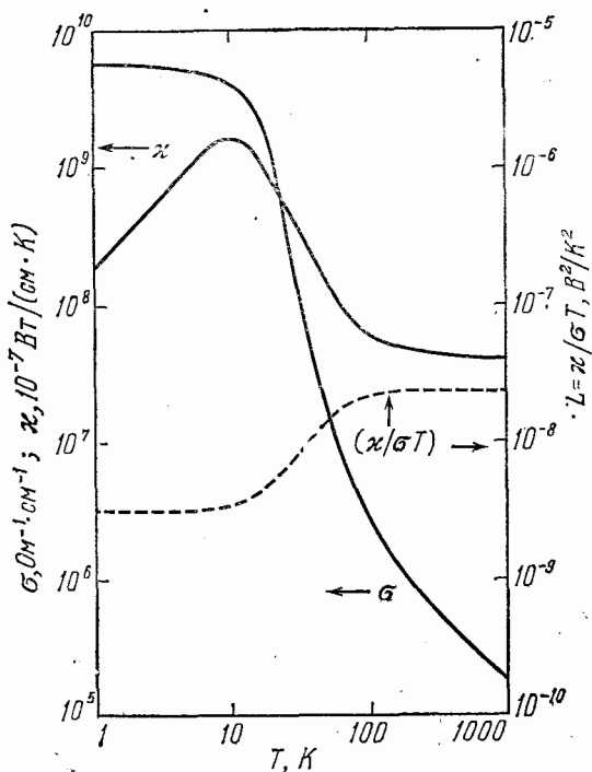
Рис. 63. Электропроводность \sigma , теплопроводность \kappa и число Лоренца L для меди. (По Блэкмору [4].)
