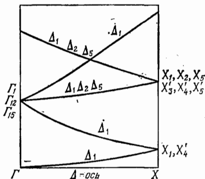
Рис. 108. Пересечение зон свободных электронов вдоль \Delta -оси в зоне Бриллюэна простой кубической решетки.
