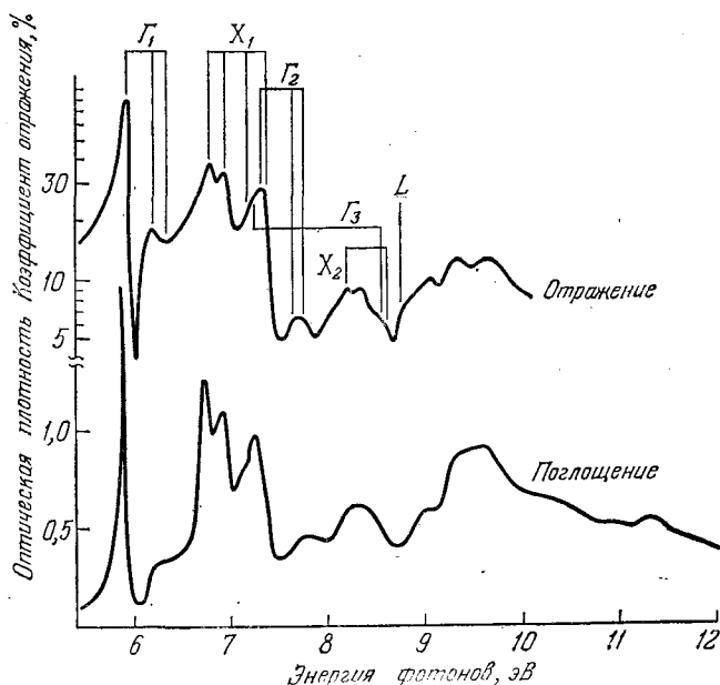
Рис. 80. Спектры отражения и поглощения KI по Балдини и Босакчи (Phys. Rev. 166 , 863, 1968), также Теегардену и Балдини (Phys. Rev. 155 , 896, 1967). Сопоставление деталей спектра отражения с переходами в зонной модели по Балдини и Босакчи там же (см. к этому рис. 79). \Gamma_1 : две экситонные линии и энергия порога для перехода из наивысшей валентной зоны в самую глубокую зону проводимости в \Gamma . X_1 : две экситонные линии и энергия порога для перехода из обеих верхних валентных зон в наиболее низкую зону проводимости в точке X . \Gamma_2 : две экситонные линии и энергия порога для переходов из более глубокой валентной зоны в нижнюю зону проводимости в \Gamma . \Gamma_3 и X_2 : экситонные линии и переходы зона—зона в более высокую зону проводимости. L : энергия порога для переходов в точке L .
