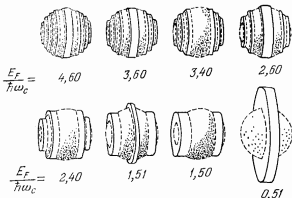
Рис 9. Состояния, распределенные в отсутствие магнитного поля равномерно в k -пространстве, в магнитном поле лежат на концентрических цилиндрах. Изображенные на рисунке цилиндрические поверхности содержат все вместе такое же число состояний, как и соответствовавшая им сфера Ферми. При слабых магнитных полях форма сферы Ферми приблизительно сохраняется. При сильных магнитных полях появляются большие отклонения. (По Адамсу и Холштейну. Не опубликовано.)
