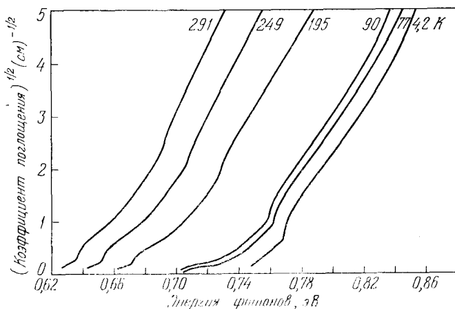
Рис. 74. Край поглощения в германии в области непрямых переходов для различных температур. (По Макферлану и др. (Phys. Rev. 108, 1377, 1957).)
