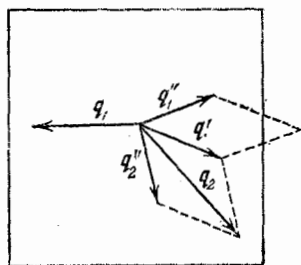
Рис. 104. Поглощение двух фононов, связанное с испусканием третьего фонона. Представлен нормальный процесс и процесс переброса.
