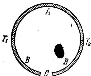
Рис. 61. Термоэлемент из двух материалов A и B с различными значениями коэффициента \epsilon .
