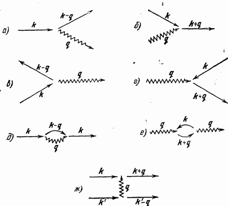
Рис. 57. Диаграммы электрон-фононного взаимодействия (процессы переброса, при которых электрон дополнительно испытывает брэгговское отражение, здесь не учитываются, см. рис. 58). а) Испускание фонона; б) поглощение фонона; в) рекомбинация электронно-дырочной пары с испусканием фонона; г) образование электронно-дырочной пары посредством фонона; д) эмиссия и реабсорбция одного (виртуального) фонона; е) превращение фонона в (виртуальную) электронно-дырочную пару; ж) электрон-электронное взаимодействие посредством обмена (виртуальным) фононом.
