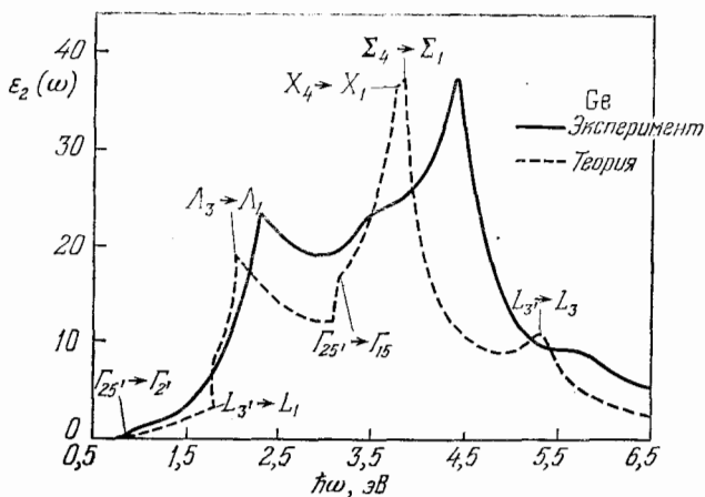
Рис. 78. Теоретический \epsilon_2 -спектр германия, сопоставленный с критическими точками перехода в зонной модели. (По Филиппсу [57. 18].)
