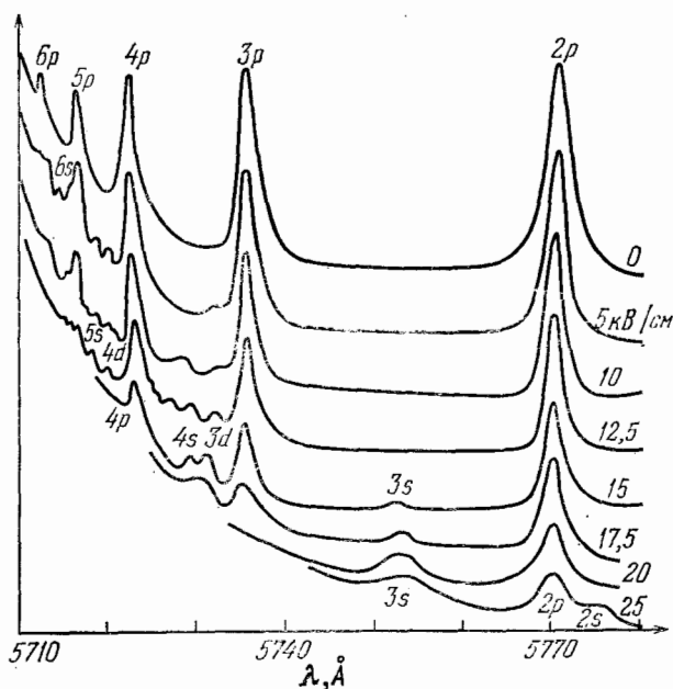
Рис. 76. Экситонные линии в \text{Si}_2\text{O} . Обозначенный на верхнем рисунке через Y дискретный спектр нанесен в измененном виде еще раз на нижнем рисунке. Как следует из правил отбора, реализуются только p -экситонные линии. Если нарушить симметрию посредством электрического поля, то окажутся возможными и s -экситонные переходы. (По Гросману [39].)
