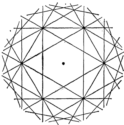
Рис. 20. Зона Бриллюэна для гексагональной плоской решетки.
