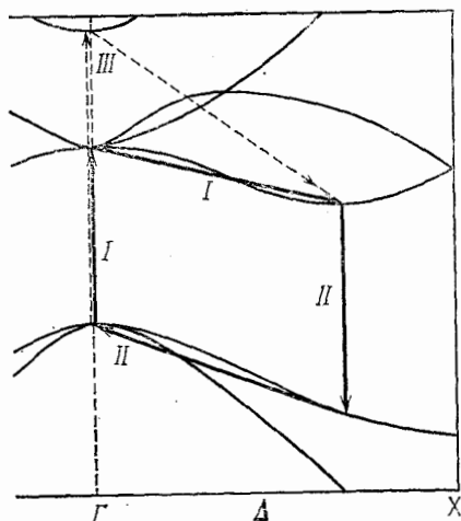
Рис. 73. Непрямые переходы в зонной структуре кремния (см. рис. 37). I: переход электрона, связанный с поглощением фотона, из валентной зоны в зону проводимости и следующий за ним переход внутри зоны проводимости при поглощении или испускании фотона. II: переход дырки, связанный с поглощением фотона, из зоны проводимости в валентную зону и следующий за ним переход дырки внутри валентной зоны при поглощении или испускании фотона. Переходы при участии более высоких зон (III) возможны, но приносят мало в поглощение.
