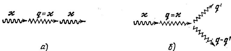
Рис. 67. Поглощение фотона, связанное с испусканием фонона: а) в последующем процессе фотон реэммитируется, б) в последующем процессе фонон распадается на два фонона меньшей энергии; только в результате этого энергия фотона окончательно извлекается из поля излучения.
